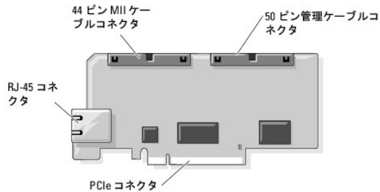
図 1-1 DRAC 5 ハードウェア機能
